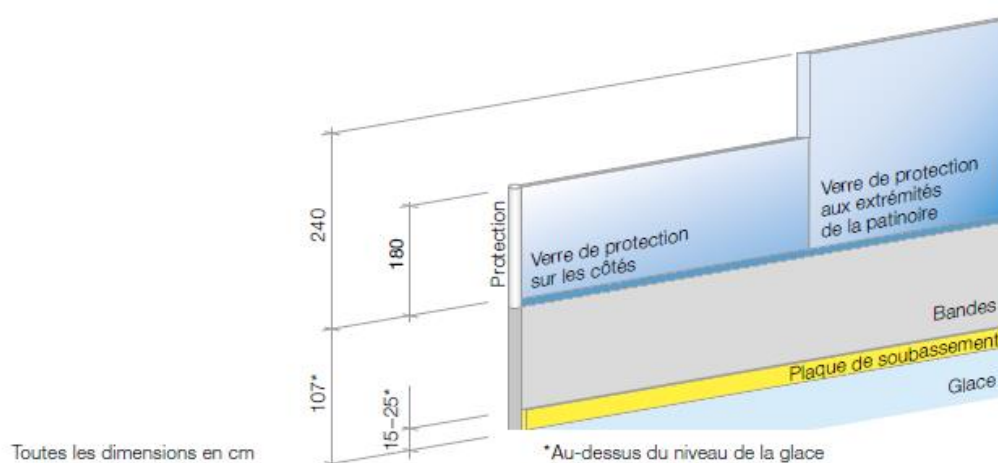
Protection types de compétitions internationales pour patinoires construites après 2015
